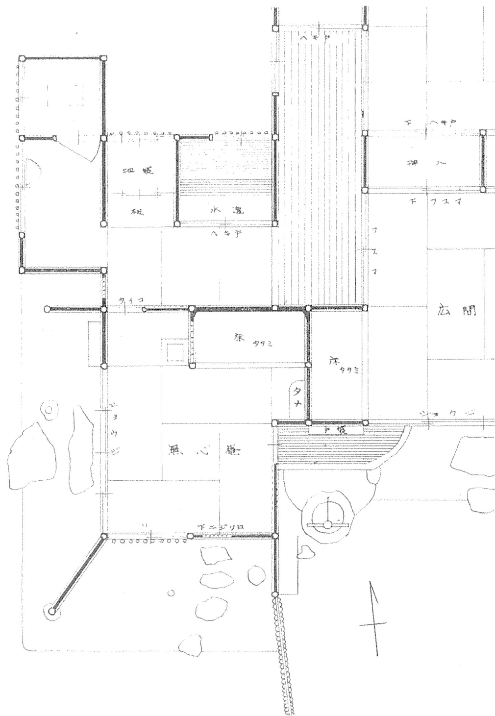
無心庵平面図
