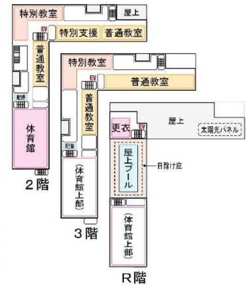
D案(北西側配置 L 字型・3階建)
