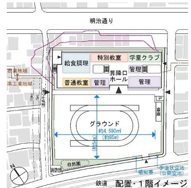
C案(北側配置 I字型・4階建)
