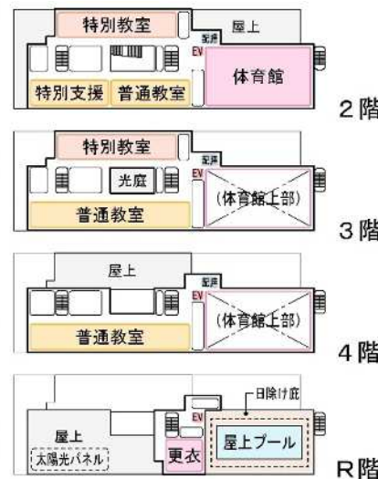
C-2案(北側配置 I 字型・4階建)
