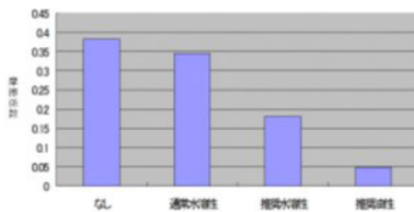
摩擦係数測定結果
