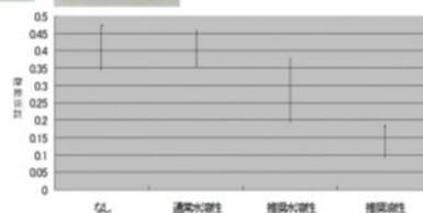
多数回振動試験結果
