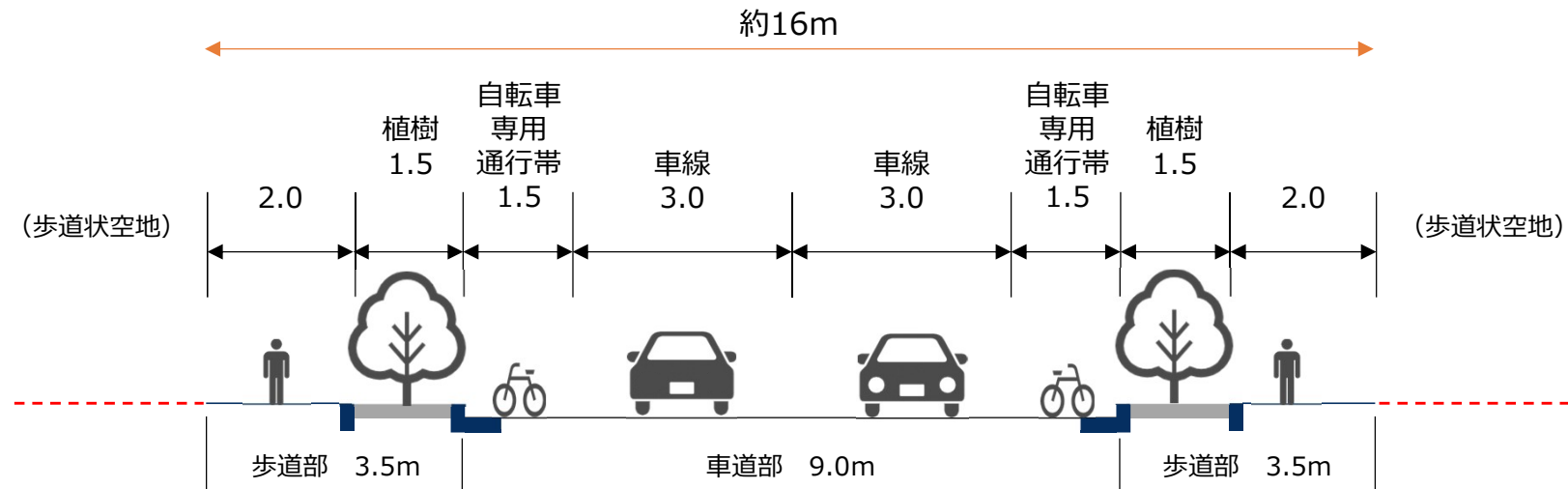
一般部の横断構成（案）
