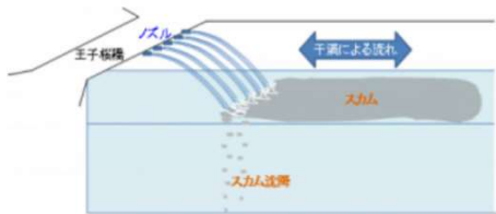
散水による打ち落としのイメージ
