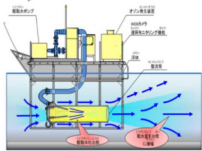
水流発生装置概略図
