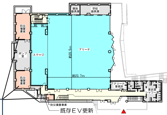
地下2階平面図
